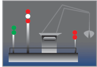
Ruoppaaja (vedenalaista työtä tekevä alus; huom. valotunnukset miltä puolelta alus on ohitettava).
