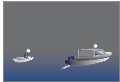
Alle 7 m pitkä konelautus voi näyttää ympäri näköpiirin näkyvää valkoista valoa.
